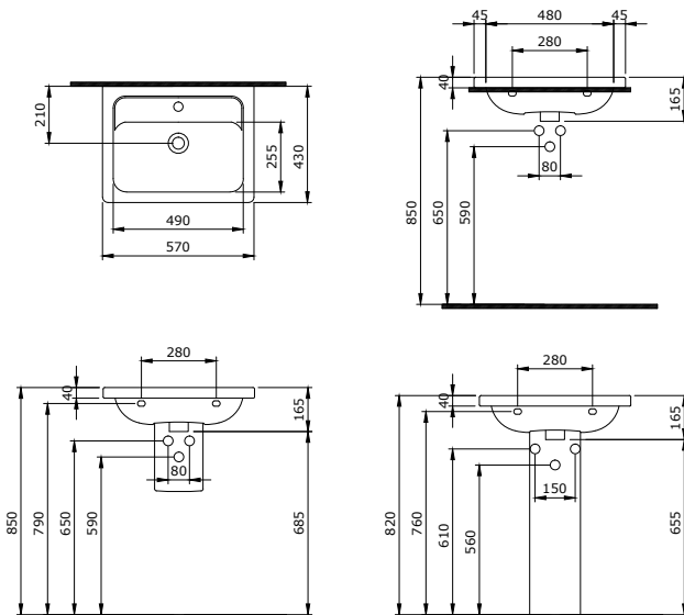
1004-001-0126 Taormina Pro Lavabo 57 cm Taormina Pro Washbasin 57 cm Taormina Pro Lavabo 57 cm
