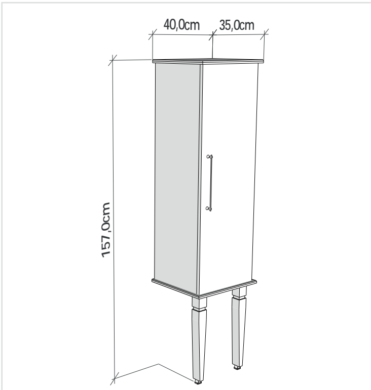
TRACE Boy dolabı Tall cabinet
