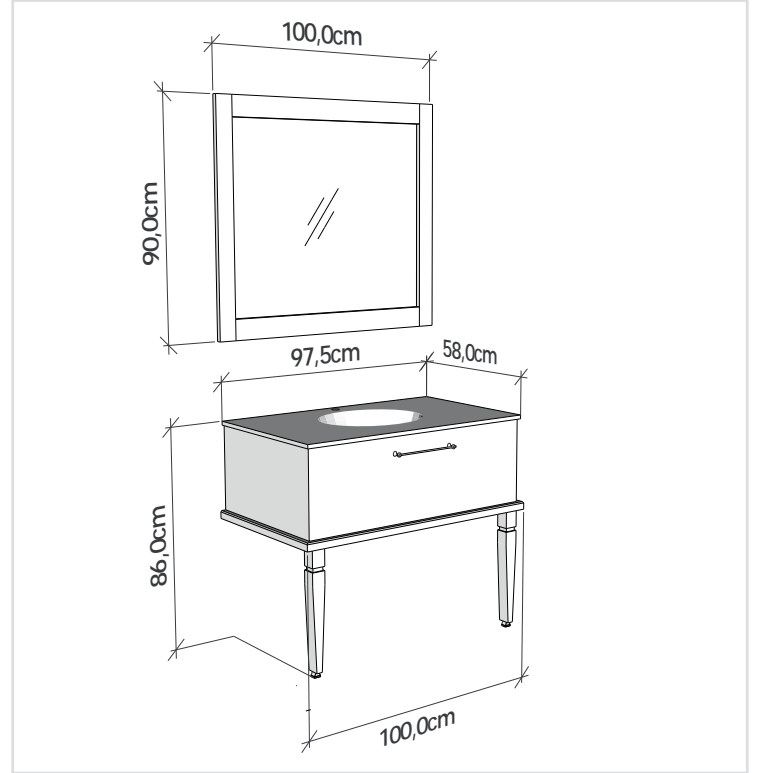
TRACE 100 cm Aydınlatmasız ayna. Mirror without illumination.
