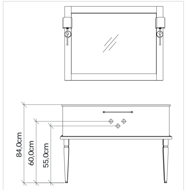
TRACE Su tesisatı ölçüsü Water installation dimension
