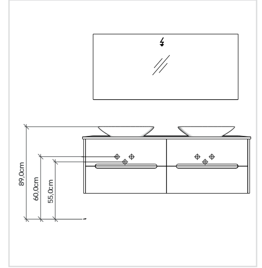
ARCADIA 14500 Su tesisatı ölçüsü Water installation dimension
